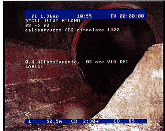
Fotografia: 1_1_6_19112012_105734_A.JPG 52,57m, 0,4 Allacciamento, 03 ore VIA DEI LARICI
